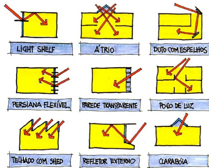
Figura 4. Sistemas de Iluminação Natural
